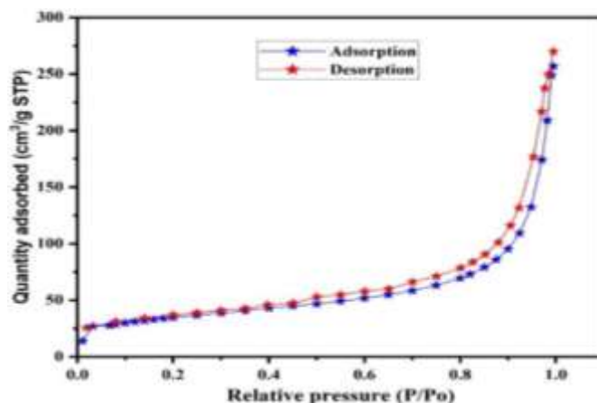
شکل ۲. ایزوترم BET نمونه گرافن اکسید-باسورین
