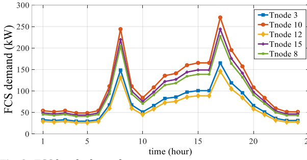
Fig. 6 : FCS hourly demand
