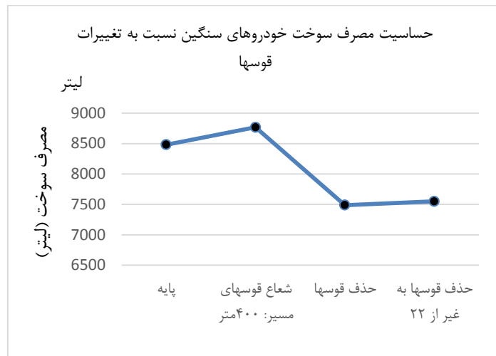
شکل ۳- نمودارهای حساسیت مصرف سوخت نسبت به تغییرات در قوس‌های مسیر
