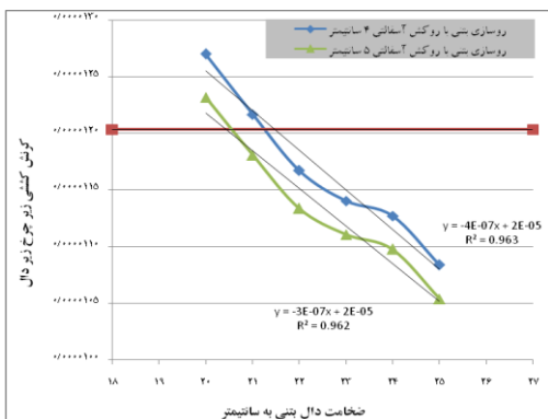
شکل ۱۰. تغییرات کرنش زیر دال با افزایش ضخامت بتن به
