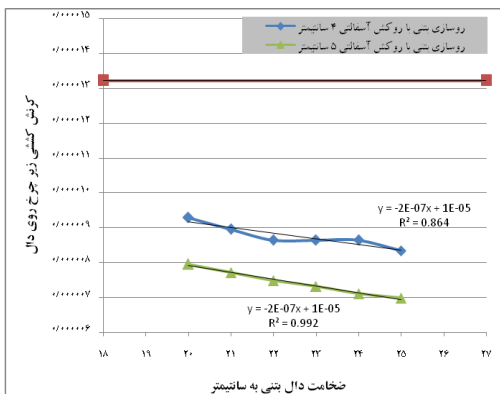
شکل ۹. تغییرات کرنش روی دال با افزایش ضخامت بتن به همراه
