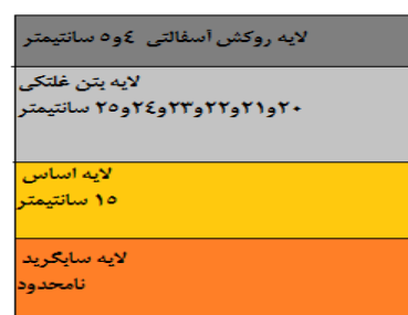
ب- روسازی بتنی با روکش آسفالت
