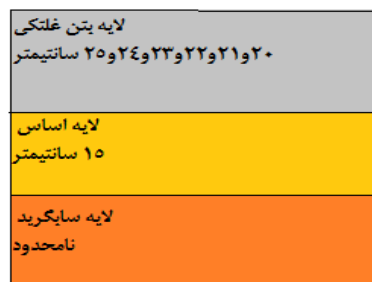
الف- روسازی بتنی
