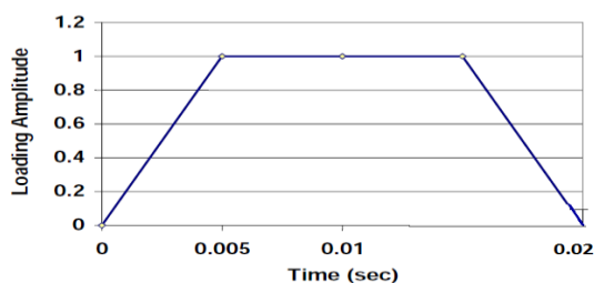
شکل ۵. دامنه بارگذاری در مدل
