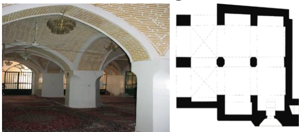
تصاویر ۱۸ و ۱۹- پلان و نمای داخلی از مسجد موسی ابن جعفر. منبع: (نگارندگان)
