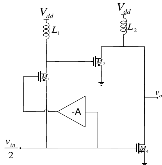
شکل ۳- ساختار ساده شده تقویت کننده پیشنهادی
