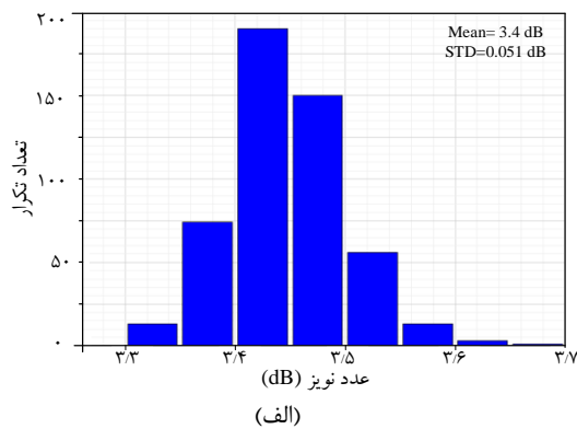
شکل ۱۹- عملکرد عدد نویز مدار در ولتاژهای تغذیه ۰/۷۵ و ۰/۸۵ ولت.
