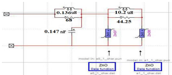
شکل (۶): مدل IEEE برق‌گیر پیشنهادی برای مطالعات [۱۶].
