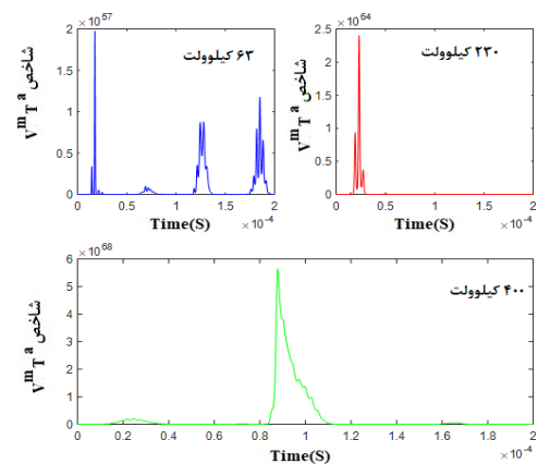
شکل (۲۱): نمودار شاخص V^{mTa} برای شکل (۱۱)
