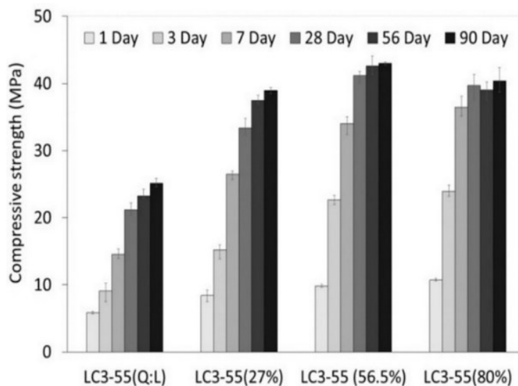
شکل ۴. تأثیر محتوای کائولینیت خاک رس کلسینه‌شده (۲۷٪، ۵۶٪، ۸۰٪) بر مقاومت فشاری (کریشان و بیشنوی، ۲۰۲۰)
