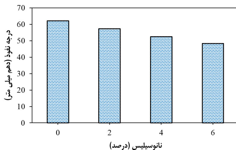
شکل ۶. تأثیر نانوسیلیس بر درجه نفوذ قیر
