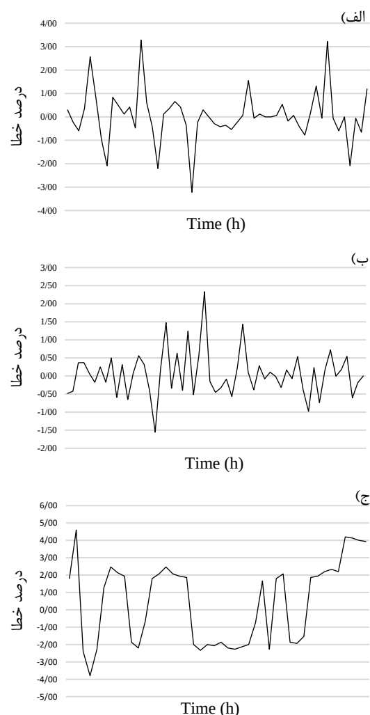
شکل ۶- نمودار خطای بهینه مدل‌ها به صورت درصدی از میانگین مقادیر مشاهداتی (الف) مدل برنامه‌نویسی بیان ژن (ب) مدل ماشین بردار پشتیبان (ج) روش سوان
