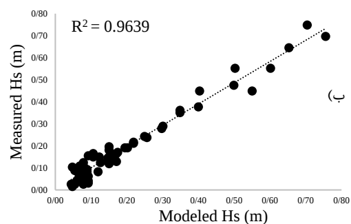
شکل ۴- پراکنش بین مقادیر اندازه‌گیری شده و مقادیر مدل‌سازی شده ارتفاع موج مشخصه الف) مدل GEP ب) مدل SVM
