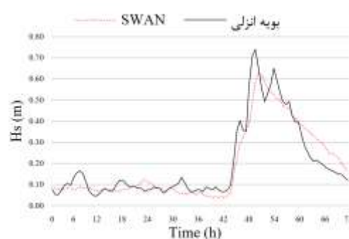
شکل ۳- سری زمانی ارتفاع موج مشخصه برای دوره صحت‌سنجی بین مقادیر اندازه‌گیری شده و مدل سوان
