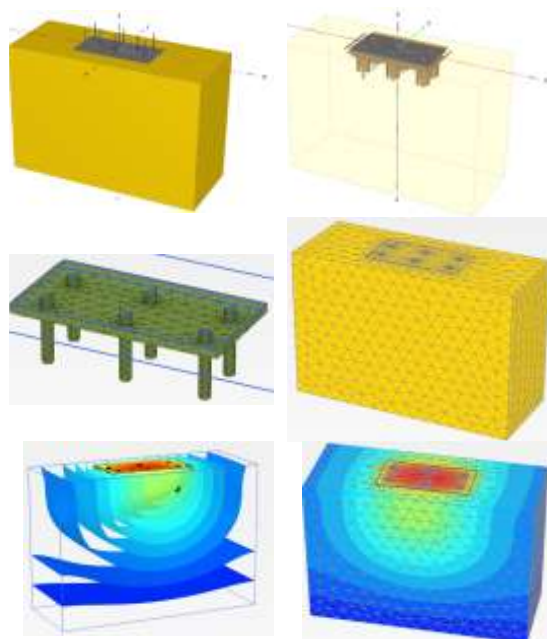
شکل ۲- مراحل شبیه سازی عددی یک نمونه از داده های تجربی یوسفی و همکاران [۲۲]، در نرم افزار المان محدود Plaxis 3D [۲۳]
