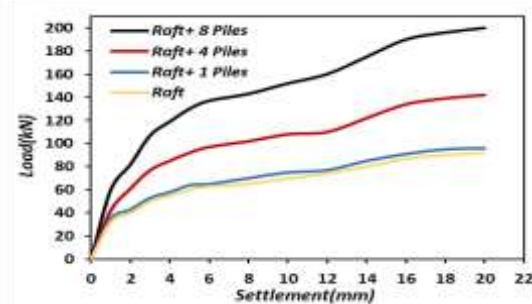
شکل ۱۰- تأثیر تعداد شمع ها بر رفتار بار-نشست برای یک نسبت معین از سختی رافت-خاک
