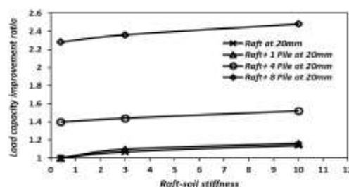
شکل ۷- تغییر نسبت بهبود ظرفیت باربری با افزایش سختی رافت-خاک برای رافت غیر مسلح و مسلح به شمع های ۱، ۴ و ۸ تایی در نشست ۲۰ میلی متر
