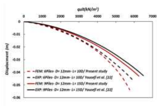
شکل ۳- مقایسه نمودار تغییرات ظرفیت باربری ( q_{ult} ) بر حسب جابجایی قائم ( \Delta ) دو نمونه تجربی یوسفی و همکاران [۲۲]، با مدل های عددی المان محدود متناظر
