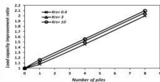
شکل ۱۱- تغییر نسبت بهبود ظرفیت باربری با افزایش تعداد شمع ها در نشست ۲۰ میلی متر برای سختی های مختلف رافت-خاک
