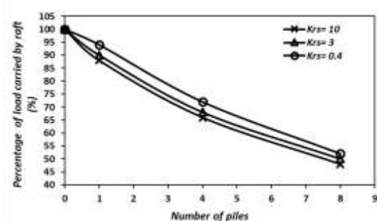
شکل ۱۳- تأثیر تعداد شمع ها بر سهم بار بین رافت و شمع برای سختی های مختلف رافت-خاک
