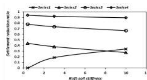
شکل ۸- تغییر نسبت کاهش نشست با سختی رافت-خاک برای رافت غیر مسلح و مسلح به شمع های ۱، ۴ و ۸ تایی
