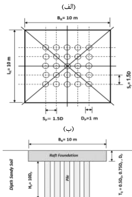
شکل ۴ - سیستم فونداسیون رافت شمعی (الف) پلان افقی (ب) نمای جانبی
