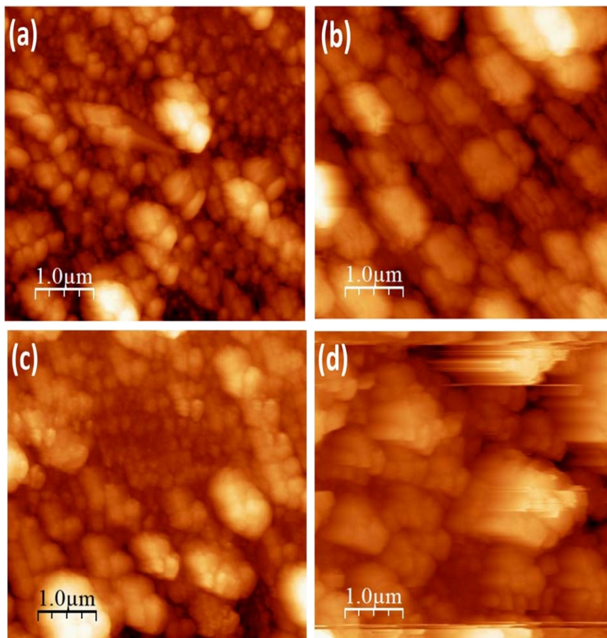
Fig. 8. AFM images of PbS nanostructures for varying film deposition time (a) 20 min, (b) 30 min, (c) 40 min, and (d) 50 min
