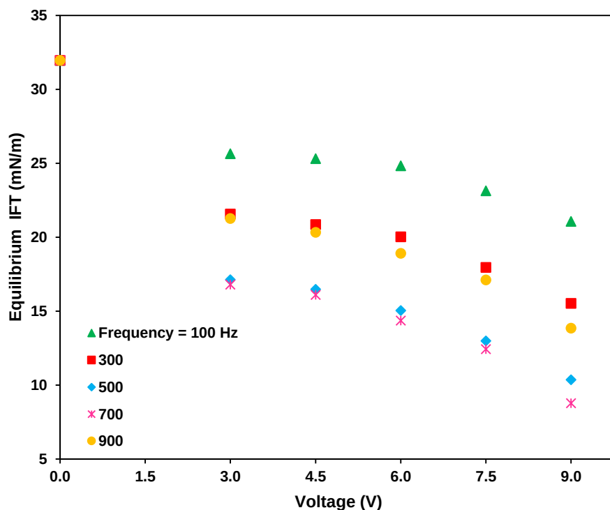
شکل ۶ تغییرات کشش بین سطحی سیستم نفت خام-آب در فرکانس‌های مختلف ولتاژ میدان الکتریکی.
