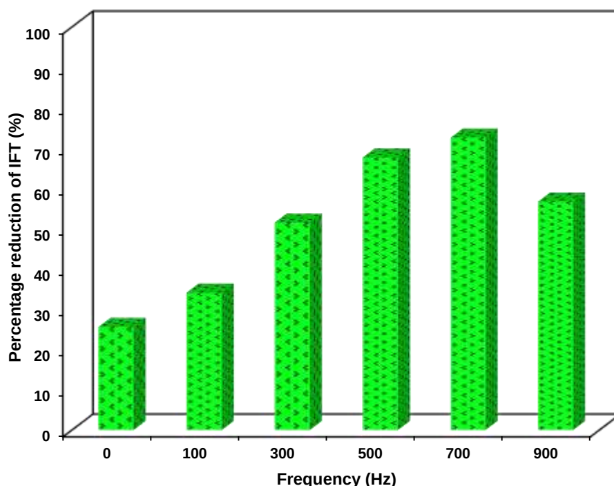
شکل ۹. تغییرات درصد کاهش کشش بین سطحی سیستم نفت خام-آب با فرکانس میدان الکتریکی نوسانی تحت ولتاژ بیشینه ۷ V.
