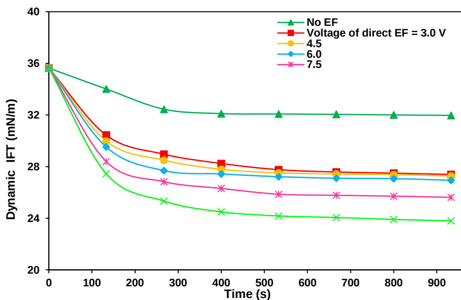
شکل ۵. تغییرات کشش بین سطحی دینامیکی سیستم نفت خام-آب برحسب زمان در ولتاژهای مختلف میدان الکتریکی مستقیم.
