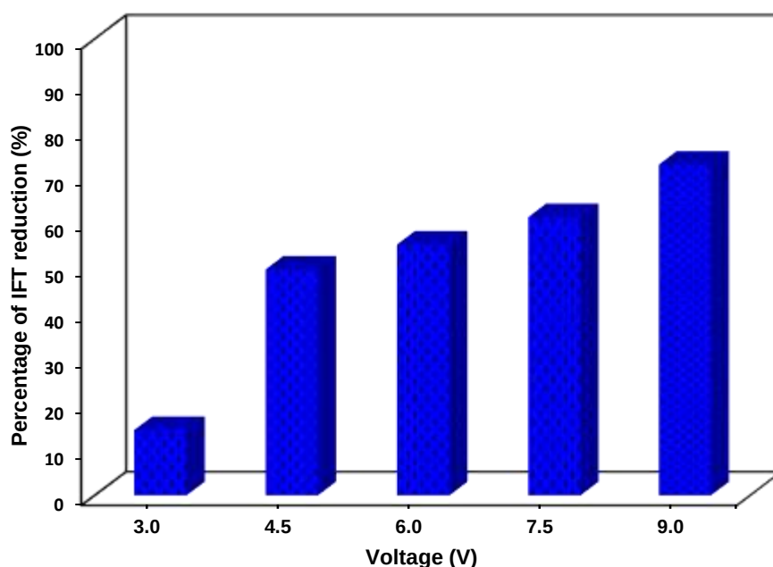
شکل ۷. نحوه تغییر درصد کاهش کشش بین سطحی سیستم نفت خام-آب با ولتاژ میدان الکتریکی نوسانی تحت فرکانس ثابت ۷۰۰ Hz.
