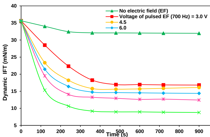
شکل ۴. تغییرات کشش بین سطحی دینامیکی سیستم نفت خام-آب برحسب زمان در ولتاژهای مختلف میدان الکتریکی نوسانی تحت فرکانس بهینه ۷۰۰ Hz.
