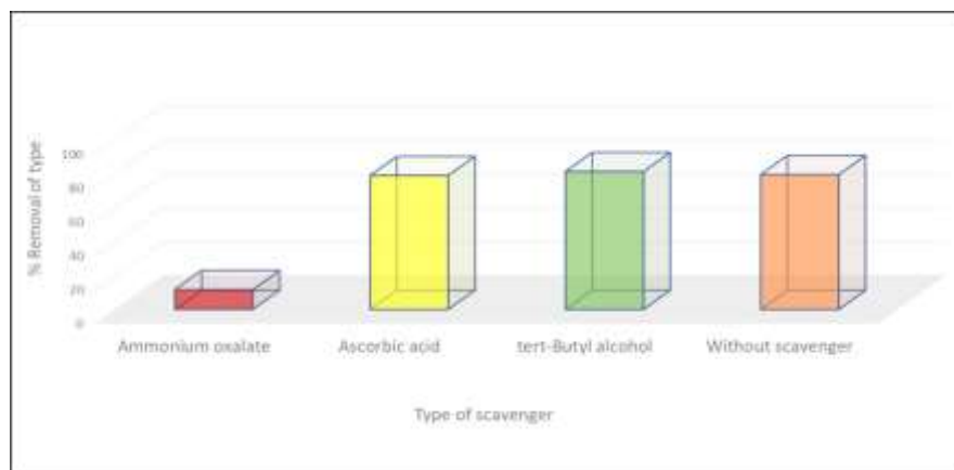
شکل ۳-۹. تأثیر بازدارنده‌های آمونیوم اگزالات (AA)، ترشیو بوتیل الکل (t-BA) و آسکوربیک اسید (AA) به ترتیب برای گونه‌های فعال حفره، رادیکال هیدروکسیل و رادیکال آنیون سوپراکسید
