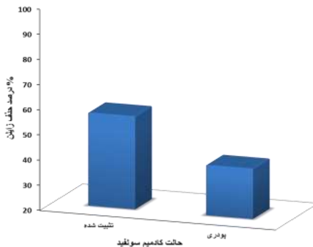
شکل ۴- درصد حذف بخارات زاین توسط کادمیم سولفید تحت تشعشع نور فرابنفش (غلظت زاین: ۳۰۰ ppm، مقدار فوتوکاتالیست: ۰/۱ g، زمان تست: ۷ ساعت)
