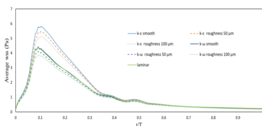
شکل ۵- نمودار تغییرات در مقادیر متوسط تنش برشی دیوار در یک سیکل قلبی
