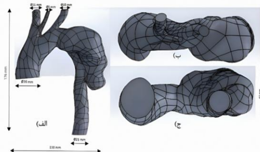
شکل ۲- مدل هندسی تولید شده (الف نمای کنار، ب نمای بالا و ج نمای زیرین)
