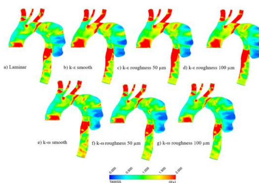
شکل ۶- تنش برشی دیواره با میانگین زمانی (TAWSS) در یک سیکل قلبی
