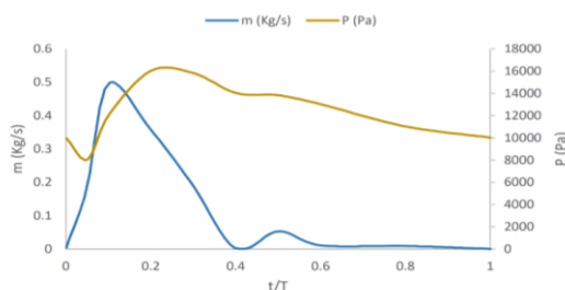
شکل ۴- شرایط مرزی ورودی (سرعت جریان جرمی) و خروجی ها (فشار)
