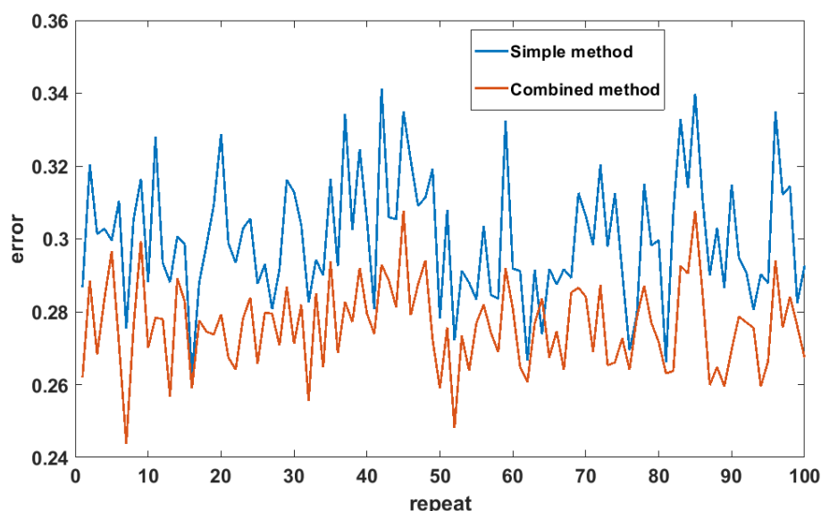
شکل ۱۰- میزان خطای محاسبه انرژی نویز به روش ساده و ترکیبی
