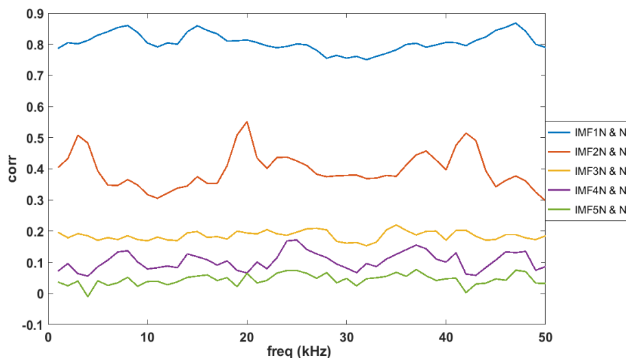
شکل ۳- میزان همبستگی به ازای نویز با واریانس کم
