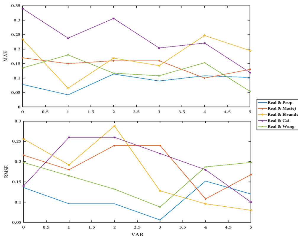
شکل ۱۴- مقایسه مقدار خطای چند روش ذکر شده با معیارهای مختلف به ازای تغییرات واریانس نویز
