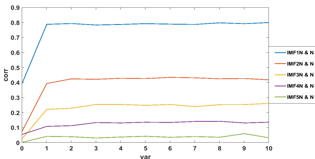
شکل ۶- میزان همبستگی به ازای سیگنال نویزی با طیف بالا
