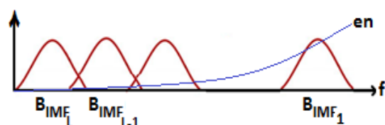
شکل ۲- تفکیک پذیری باندهای فرکانسی لایه‌ها و انرژی نویز
