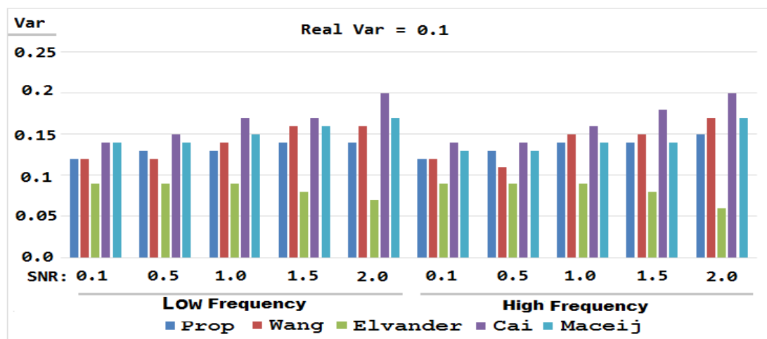
شکل ۱۶- مقایسه مقدار واریانس تخمینی روش پیشنهادی با روش‌های موجود به ازای \text{var}=0.1 و تغییرات فرکانس و SNR
