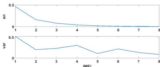
شکل ۱۱- نمودار انرژی نویز و واریانس لایه‌های تجزیه شده
