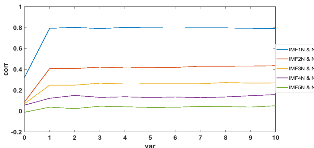
شکل ۵- میزان همبستگی به ازای سیگنال نویزی با طیف پایین
