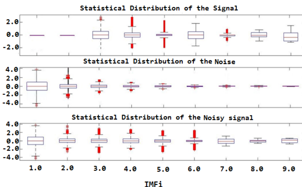
شکل ۱۲- توزیع آماری از سیگنال، نویز و سیگنال نویزی
