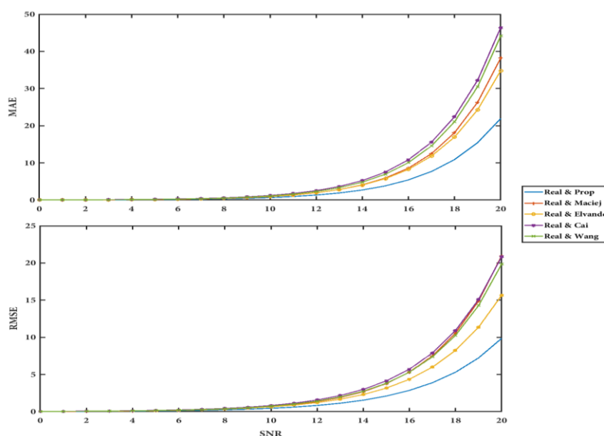
شکل ۱۵- مقایسه مقدار خطای چند روش ذکر شده با معیارهای مختلف به ازای تغییرات SNR
