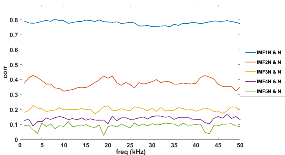
شکل ۴- میزان همبستگی به ازای نویز با واریانس زیاد
