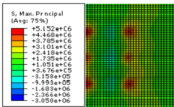
شکل ۷- توزیع تنش در زیر دال بتنی تحت بارگذاری هواپیمای B777-300ER
