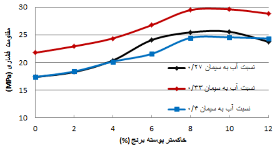
شکل ۱۲. تأثیر نسبت‌های آب به سیمان ۰/۲۷، ۰/۳۳ و ۰/۴ بر مقاومت فشاری بتن حاوی الیاف و خاکستر پوسسته برنج
