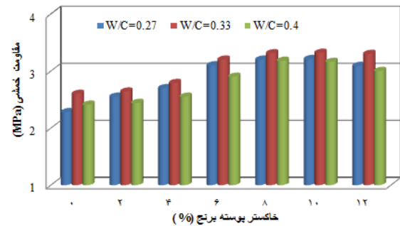
شکل ۱۱. مقاومت خمشی بتن حاوی الیاف و خاکستر پوسسته برنج در نسبت‌های آب به سیمان ۰/۲۷، ۰/۳۳، و ۰/۴
