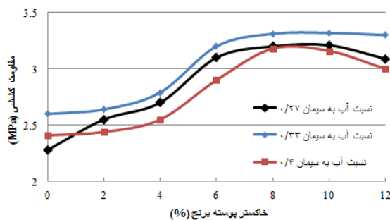
شکل ۱۳. تأثیر نسبت‌های آب به سیمان ۰/۲۷، ۰/۳۳ و ۰/۴ بر مقاومت کششی بتن حاوی الیاف و خاکستر پوسسته برنج
