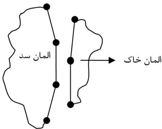
شکل ۴- گره های المان فصل مشترک خاک و سد
