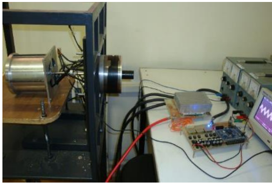
شکل ۱۰- چیدمان آزمایشگاهی
