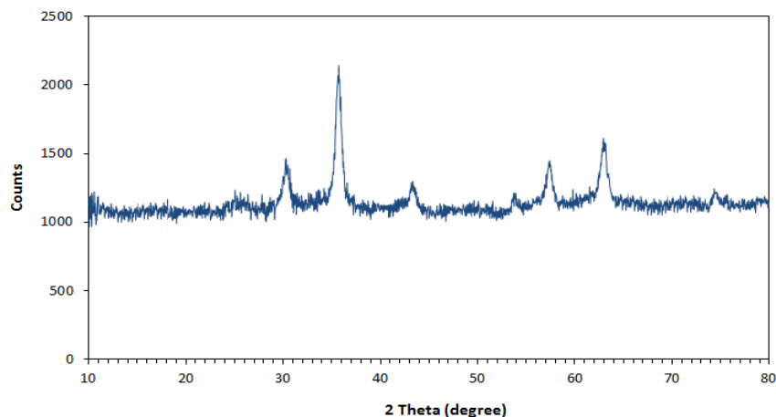
شکل ۳- طیف پراش پرتو X برای mMWCNT
