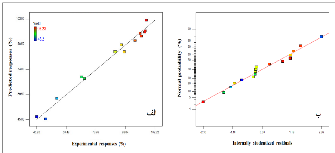
شکل ۴- الف) مقادیر پاسخ‌های پیش‌بینی شده به وسیله مدل مرتبه دوم در مقابل مقادیر تجربی، و ب) نمودار احتمال نرمال برای باقیمانده‌های برآورد شده با مدل مرتبه دوم برای حذف رنگ DG۲۶ به وسیله mMWCNT
