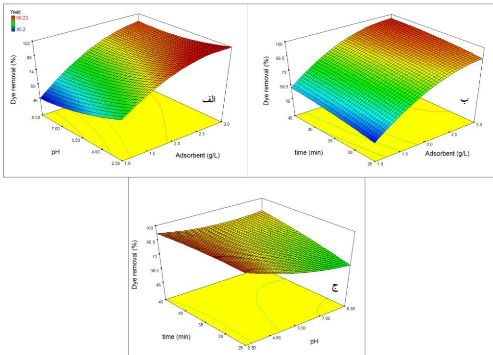
شکل ۶- نمودار سه بعدی سطح پاسخ مربوط به اثر برهم‌کنش‌های دو فاکتوری (الف) مقدار جاذب و pH، (ب) مقدار جاذب و زمان تماس، (ج) pH و زمان تماس بر درصد حذف DG۲۶ به وسیله mMWNT
