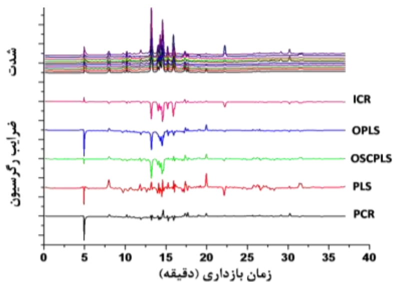
شکل ۴- کروماتوگرام‌های HPLC-DAD و نمودارهای ضریب رگرسیون به‌دست آمده از اجرای مدل‌های مختلف روی داده‌ها در عصاره گیاه گردو با غلظت ۰/۷۵ میلی‌گرم بر میلی‌لیتر با فاز متحرک استونیتریل و مخلوط آب + ۰/۱ درصد اسید فرمیک و سرعت جریان حلال ۰/۵ میلی‌لیتر بر دقیقه
