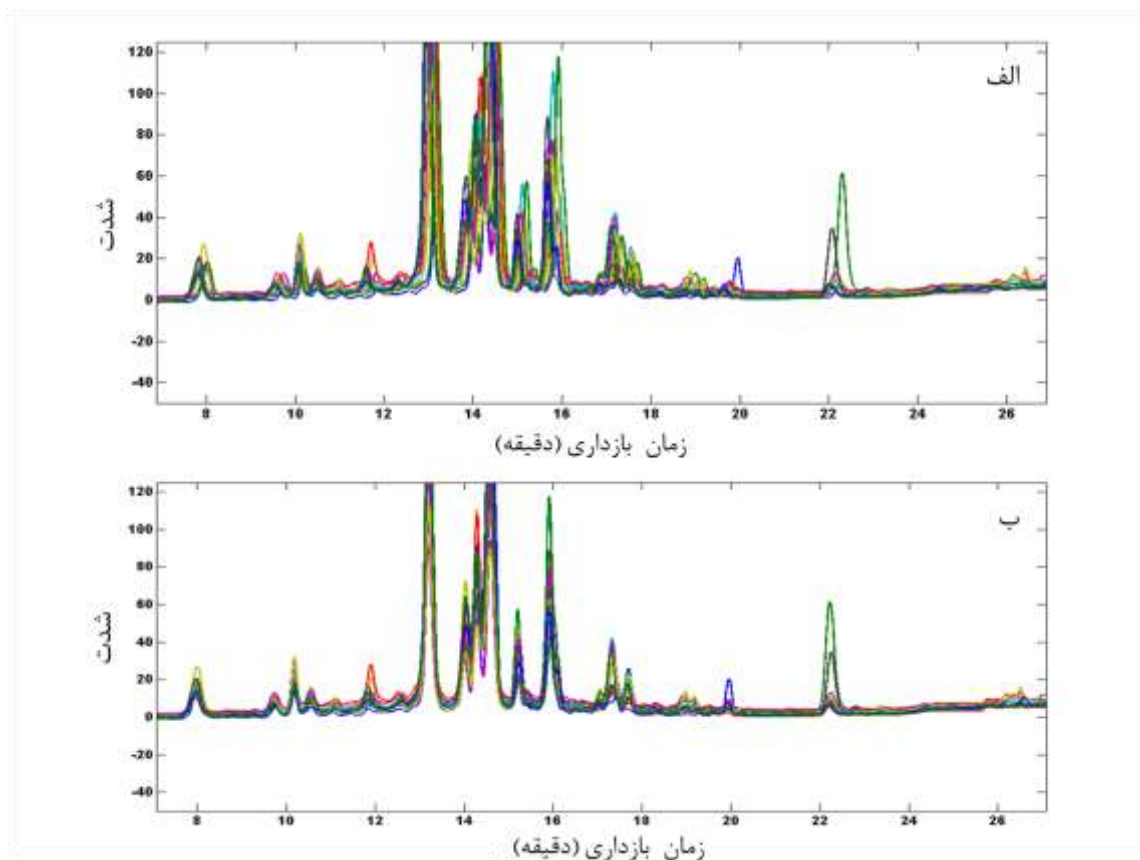
شکل ۲- محدوده‌ای از کروماتوگرام‌های نمونه‌ی برگ گردو با غلظت 0/75 میلی‌گرم بر میلی‌لیتر در طول موج 254 نانومتر، فاز متحرک استونیتریل و مخلوط آب + 0/1 درصد اسید فرمیک و سرعت جریان حلال 0/5 میلی‌لیتر بر دقیقه (الف) قبل از هم‌ترازی با COW (ب) بعد از هم‌ترازی با COW
