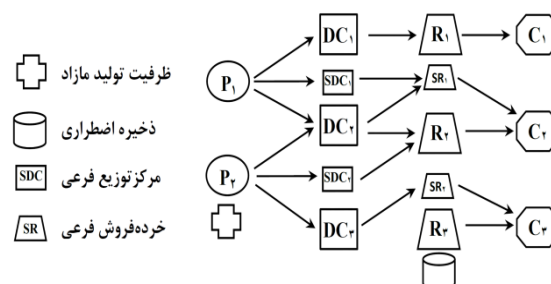
شکل ۲: ساختار شبکه زنجیره تأمین ارتجاعی
