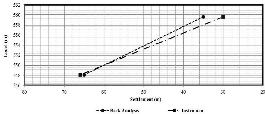
شکل ۸- مقایسه مقادیر نشست به دست آمده با استفاده از ابزار دقیق و مدل سازی عددی در بحرانی ترین مقطع سد پس از اولین دوره آبگیری.
