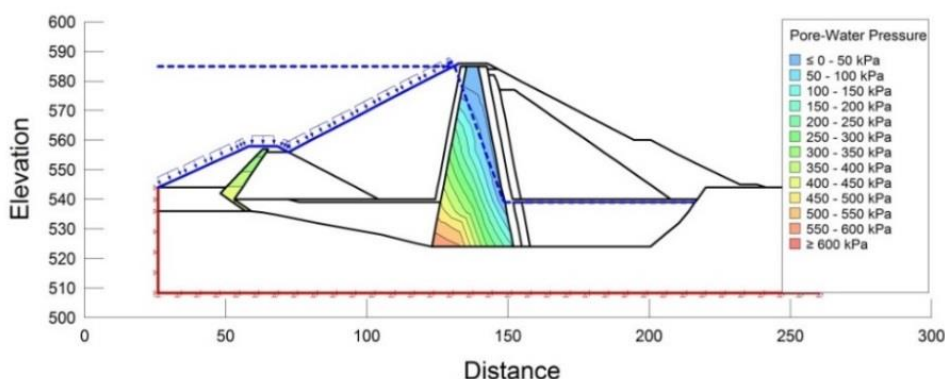
شکل ۱۵- مقادیر فشار منفذی در هسته سد در اولین مرحله آنگیری.
