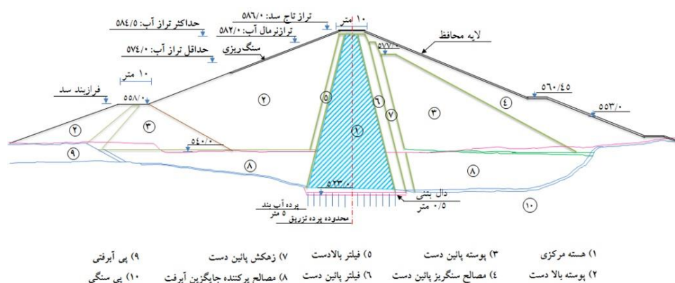
شکل ۱- مقطع عرضی سد چهچهه.
