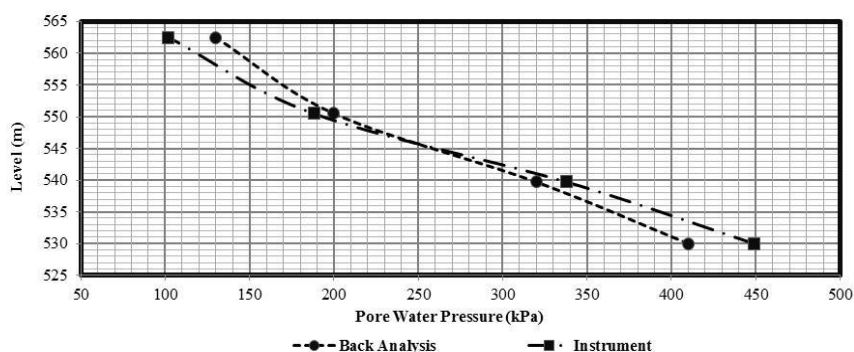
شکل ۱۶- تغییرات فشار آب منفذی در ترازهای ارتفاعی مختلف پس از اولین آنگیری با استفاده از نتایج ابزار دقیق و مدل‌سازی عددی.
