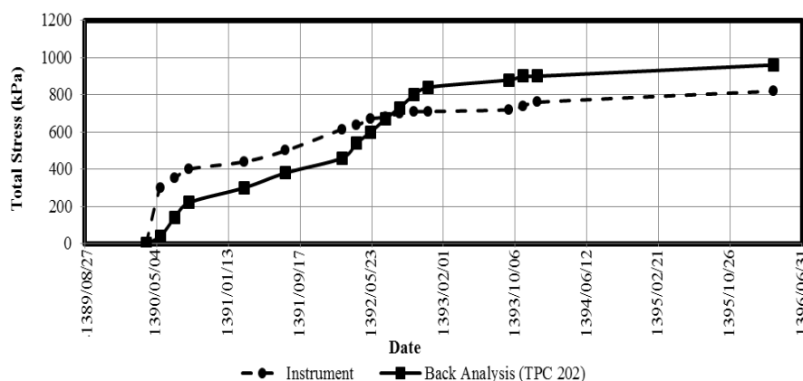
شکل ۹- تغییرات تنش کل از ابتدای ساخت تا اولین مرحله آبگیری در هسته سد با استفاده از نتایج قرائت شده سلول فشار نصب شده در تراز ۵۳۰ متری و مدل سازی عددی
