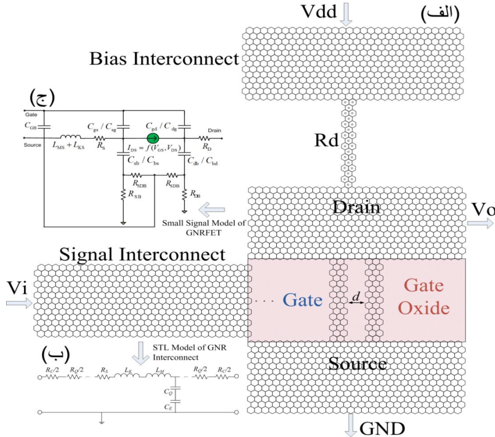
شکل ۱- (الف) ساختار پیشنهادی اینورتر گرافنی یکپارچه، (ب) مدل مداری خط ارتباطی نانونوارگرافنی، (ج) مدل مداری ترانزیستور اثر میدان نانونوار گرافنی
