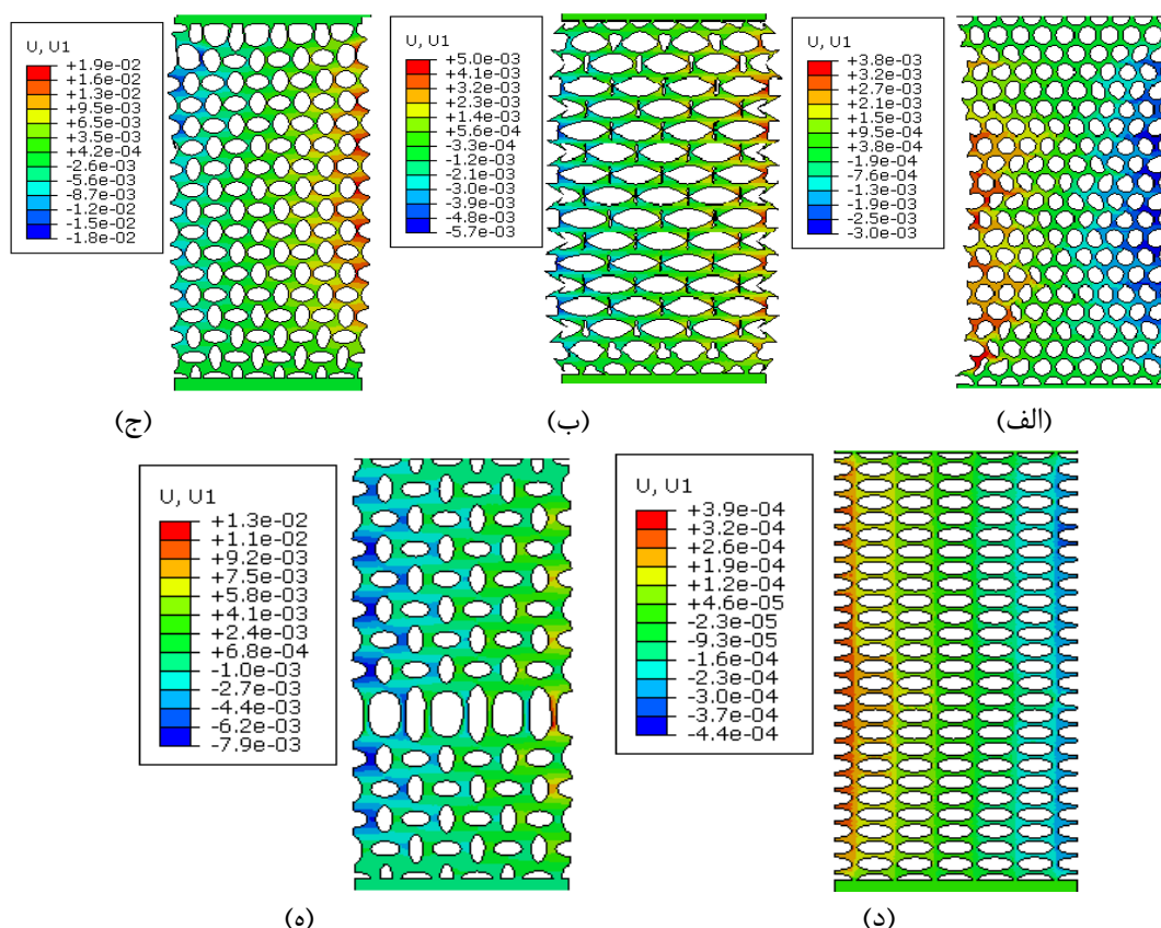
شکل ۴ مکانیزم تغییر شکل (m) تعدادی از نمونه‌های مختلف میراگر فلزی ارائه شده Type V (ه) و Type IV (د)، Type III (ج)، Type II (ب)، Type I (الف)
