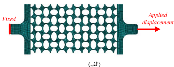
شکل ۲ میراگر فلزی جاری شونده آگرتیک جدید ارائه شده در تحقیق حاضر
