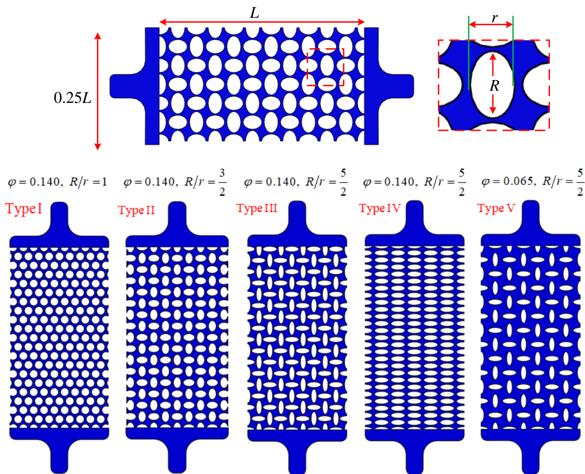
شکل ۲ میراگر فلزی جاری شونده آگرتیک جدید ارائه شده در تحقیق حاضر
