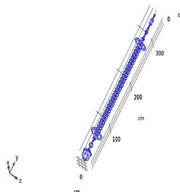
شکل ۴- مدل سه بعدی مقره کامپوزیت ۲۳۰ کیلوولت
