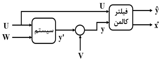
شکل ۲- ساختار کلی فیلتر کالمن برای تخمین حالت‌های یک سیستم با داشتن نویزهای فرآیند و اندازه‌گیری
