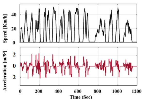
شکل ۵- الگوی حرکتی سرعت و شتاب اتوبوس برقی در خطوط شهری برای انجام محاسبات توان و انرژی [۳۰]
