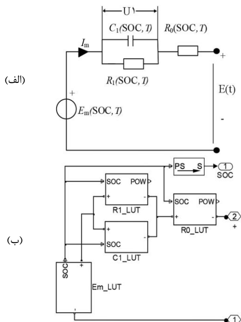
شکل ۶- الف) مدار معادل استفاده شده در این مقاله. ب) بلوک مدار معادل مرجع [۲۸] طراحی شده با بلوک‌های جدول جستجوی دو بعدی Simscape در سیمولینک متلب.
